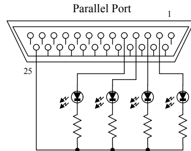
그림 2. 병렬포트에 의한 회로 Fig. 2. Circuit using Parallel Port
