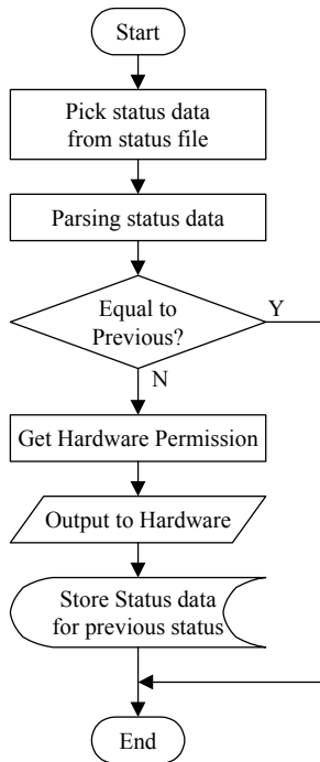
그림 3. 처리의 흐름도 Fig. 3. Flow diagram of processing
