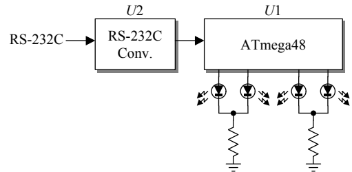
그림 4. 실험 회로의 블록도 Fig. 4. Block diagram of Experimental Circuit
