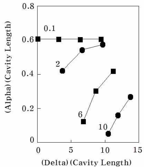
그림 2. \rho_l 의 위상= \pi/2 , \rho_r 의 위상= -\pi/2 , \delta L > 0 인 경우, \kappa L 이 증가할 때 (\alpha L, \delta L) 의 변화 그래프 Fig. 2. The graph of (\alpha L, \delta L) in case of \rho_l phase= \pi/2 , \rho_r phase= -\pi/2 , and \delta L > 0 as \kappa L increases
