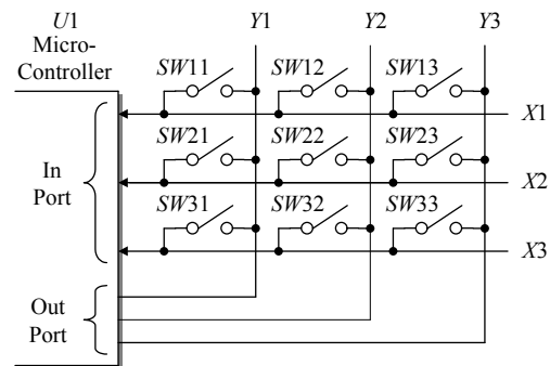
그림 1. 다이내믹 스캐닝의 예 Fig. 1. Example of the dynamic scanning
