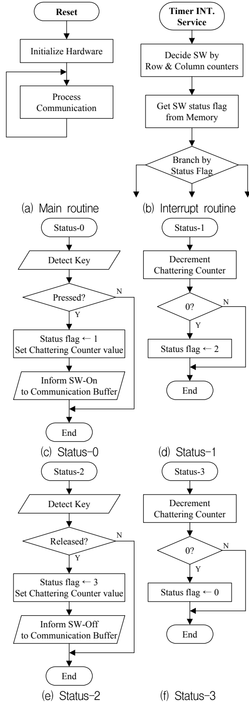
그림 6. 키의 상태별 처리 흐름도 Fig. 6. Flowchart for each key-status
