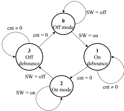
그림 5. 각 키의 처리 상태도 Fig. 5. Status diagram of each key
