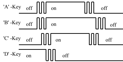
그림 3. 동시 스위치 검출의 예 Fig. 3. Example of detecting switch simultaneously
