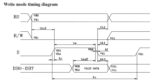
그림 3. LCD timing diagram
