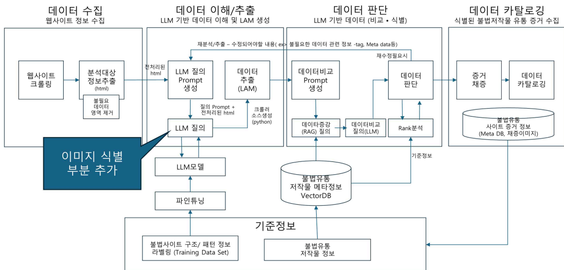
그림 2. 이미지 식별 기능이 포함된 불법 OTT 콘텐츠 탐지 및 증거 수집 시스템 아키텍처 Fig. 2. System Architecture for Illegal OTT Content Detection and Evidence Collection with Image Identification
