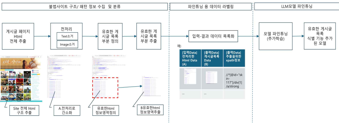
그림 4. 불법 유통 사이트 식별을 위한 학습 데이터 수집 및 LLM 모델 파인튜닝 과정 Fig. 4. Training Data Preparation and Fine-Tuning Workflow for Illegal Distribution Site Detection Using LLM
