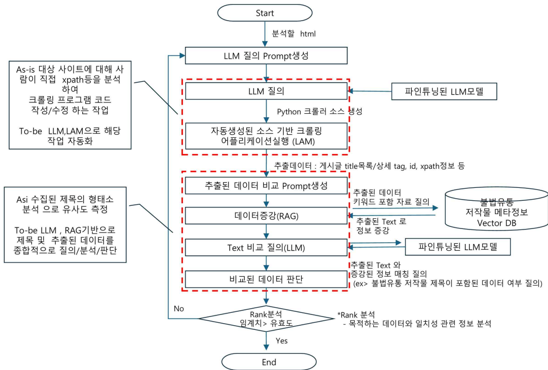
그림 3. 기존 수작업 방식 대비 LLM·LAM 기반 자동화 흐름 비교도 Fig. 3. Comparison Flow of Manual Process vs. LLM·LAM-Based Automation
