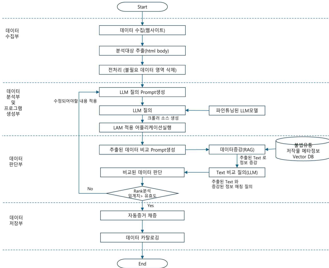
그림 1. OTT 콘텐츠 불법 유통 탐지 및 증거 수집 자동화 처리 흐름도 Fig. 1. Automated Workflow for Detecting and Collecting Evidence of Illegal OTT Content Distribution
