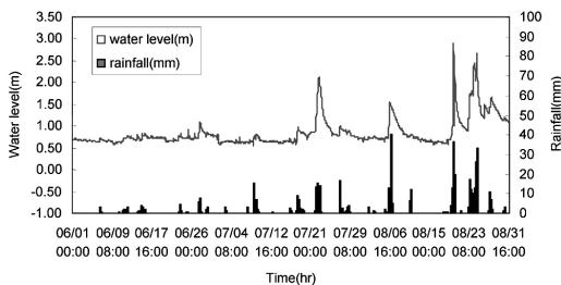
그림 4. 울문천의 수위변동(2003년 6월~8월)
