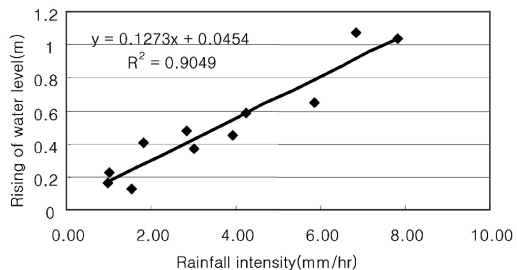
그림 8. 강우강도와 수위상승과의 관계(지암천)
