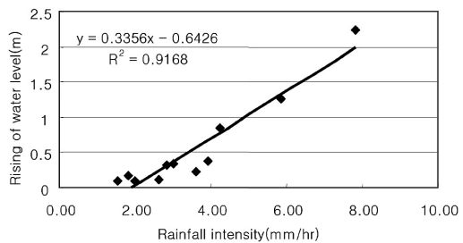
그림 7. 강우강도와 수위상승과의 관계(울문천)
