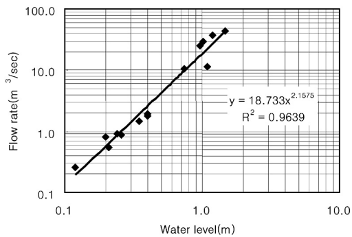
그림 9. 수위·유량 곡선(공지천)
