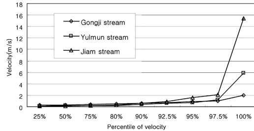
그림 12. 하천별 유속 변화
