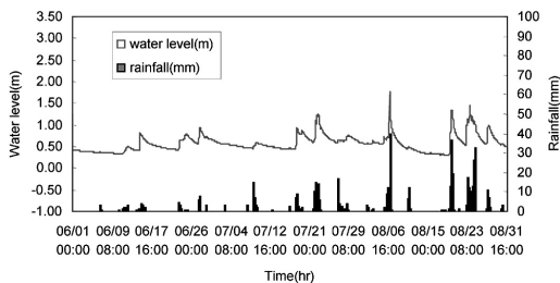
그림 5. 지암천의 수위변동(2003년 6월~8월)
