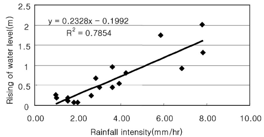
그림 6. 강우강도와 수위상승과의 관계(공지천)
