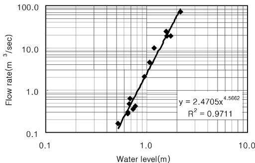
그림 10. 수위·유량 곡선(울문천)
