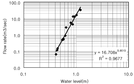
그림 11. 수위·유량 곡선(지암천)
