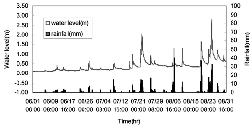
그림 3. 공지천의 수위변동(2003년 6월~8월)
