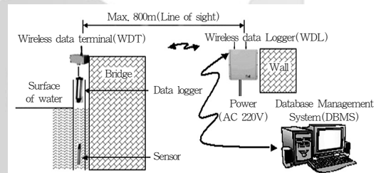
그림 1. 무선원격수위계측시스템의 구성도
