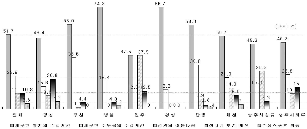
그림 6. 충주호 및 그 주변하천의 수질개선시 기대항목
