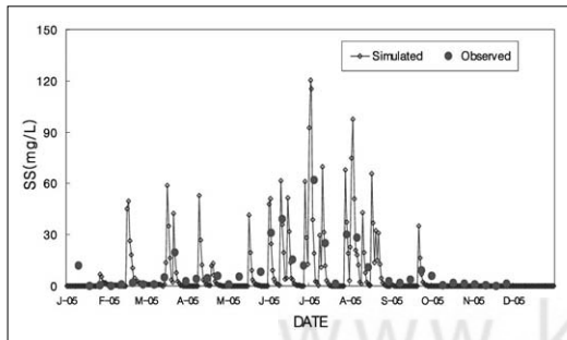
그림 13. 유사량의 검증결과
