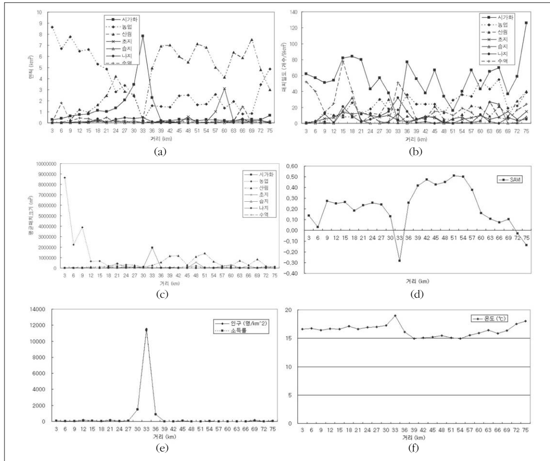
그림 5. 천안시의 단계적 변화 분석: (a) 각 토지이용의 면적, (b) 패치밀도, (c) 평균패치크기, (d) SAVI, (e) 인구밀도, 소득률, (f) 온도
