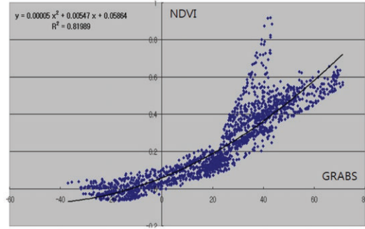
그림 8. NDVI와 GRABS 값의 산포도
