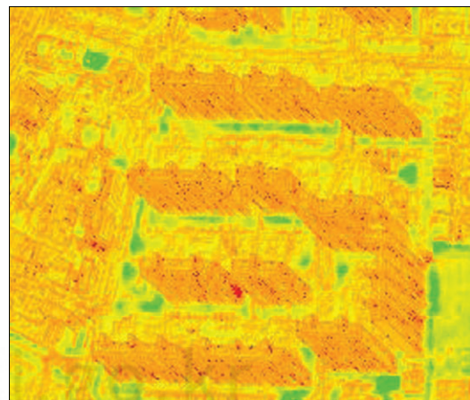
그림 10. 보정 후 NDVI값의 분포특성
