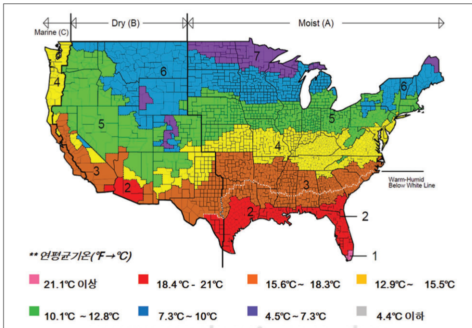
그림 2. 미국의 기후대별 Cool Roof 적용 우선 등급지도
