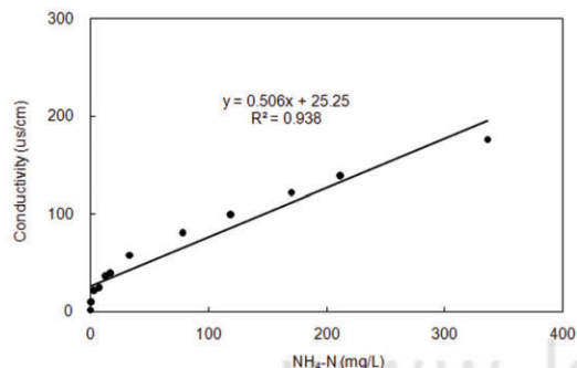
그림 5. 유입수내 NH_4-N 농도별 EC 계측 정확도 평가
