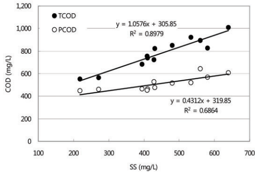
그림 4. 유입수내 COD 농도별 SS 계측 정확도 평가
