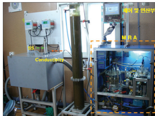
그림 2. 실시간 하수처리장 유입수 특성분석장치-MRA2
