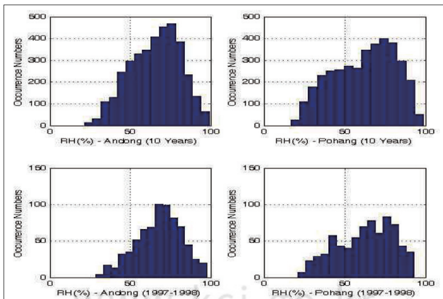
그림 5. 상대습도의 빈도분포
