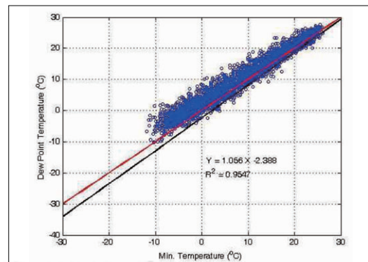
(b) 목포
