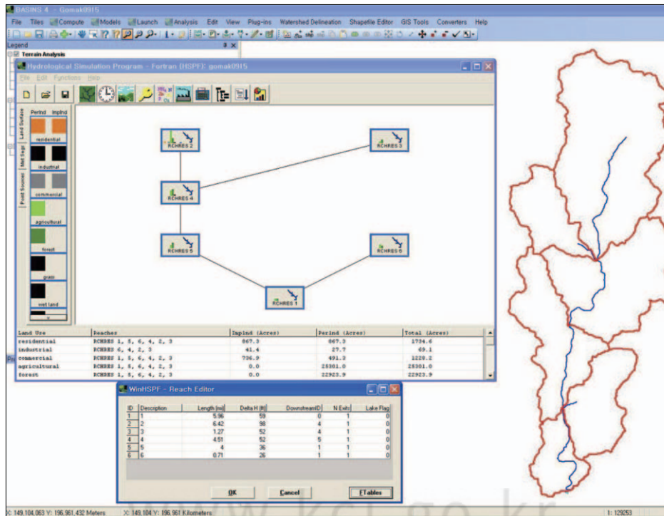
그림 5. WinHSPF reach editor
