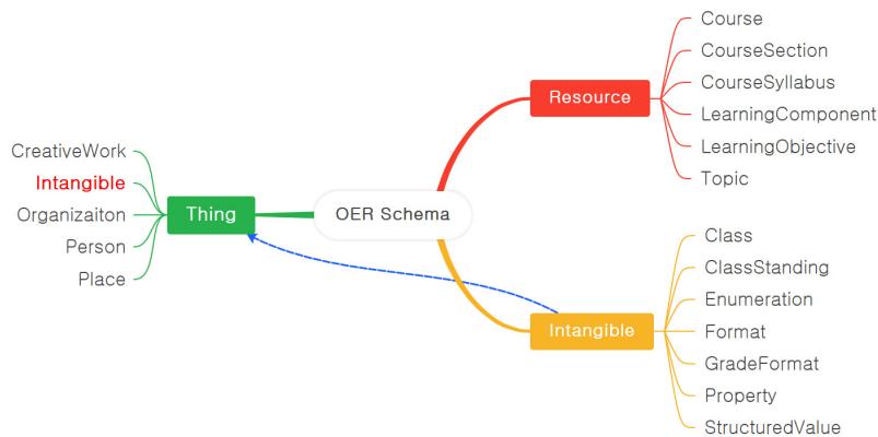
〈그림 4〉 OER Schema 타입 관계도; 2단계까지 표현
