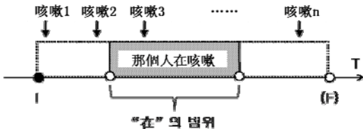
[그림2] “那個人在咳嗽”의 내부시간구조
