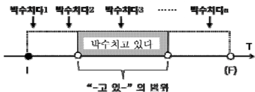
[그림3] “박수치고 있었다”의 내부시간구조 7)
