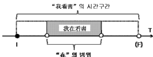
[그림1] “我在看書”의 내부시간구조
