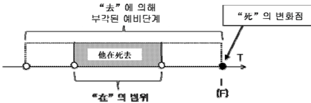
[그림5] “他在死去”의 내부시간구조
