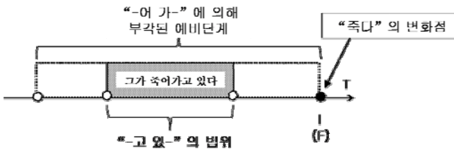
[그림4] "죽어가고 있다"의 내부시간구조
