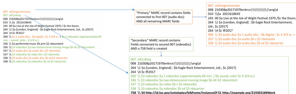
<그림 2> 007 필드와 300 필드(딸림자료)를 이용해 다수의 인스턴스 생성
