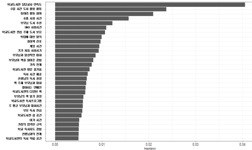
〈그림 3〉 설명변수의 중요도(Feature Importance) 결과
