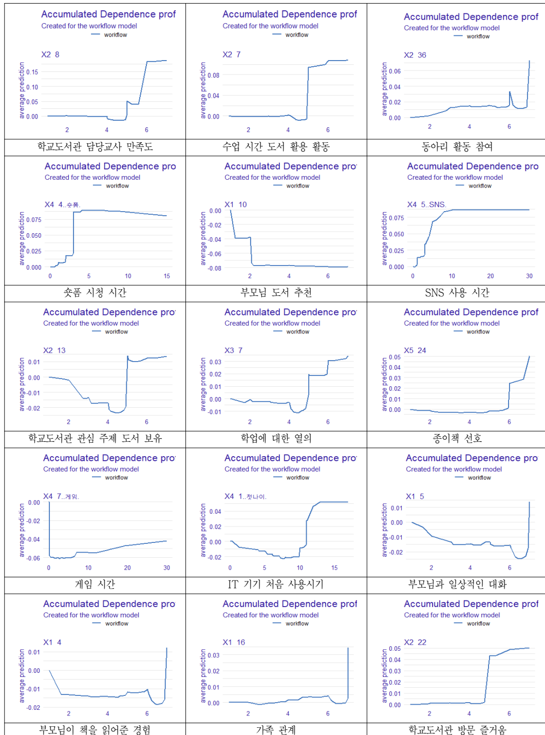
〈그림 4〉 주요 변수별 부분 의존성 도표(Partial Dependence Plot)
