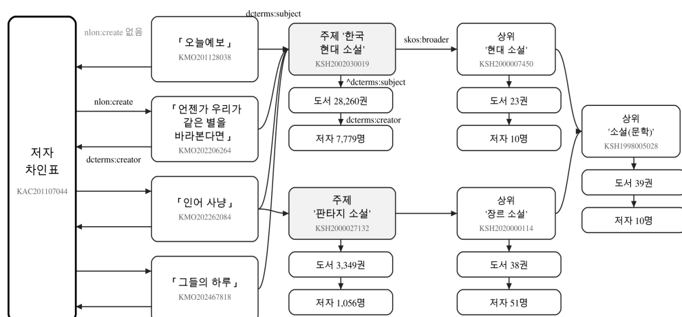
<그림 2> 연결 관계 확장의 예시
