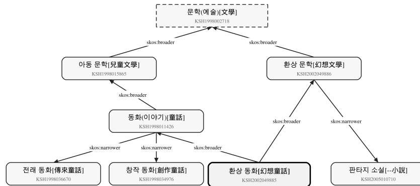
〈그림 3〉 주제 그래프의 연결 예시
