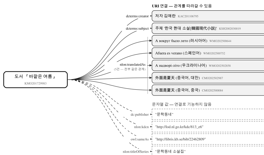
〈그림 1〉 도서 「바깥은 여름」 개체의 URI 연결과 문자열 값
